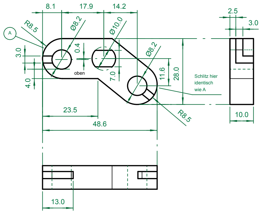
Schalthebel, Aluminium (1X)
