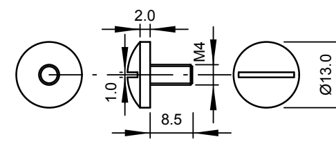
Sicherungsschraube, Stahl (1x)
