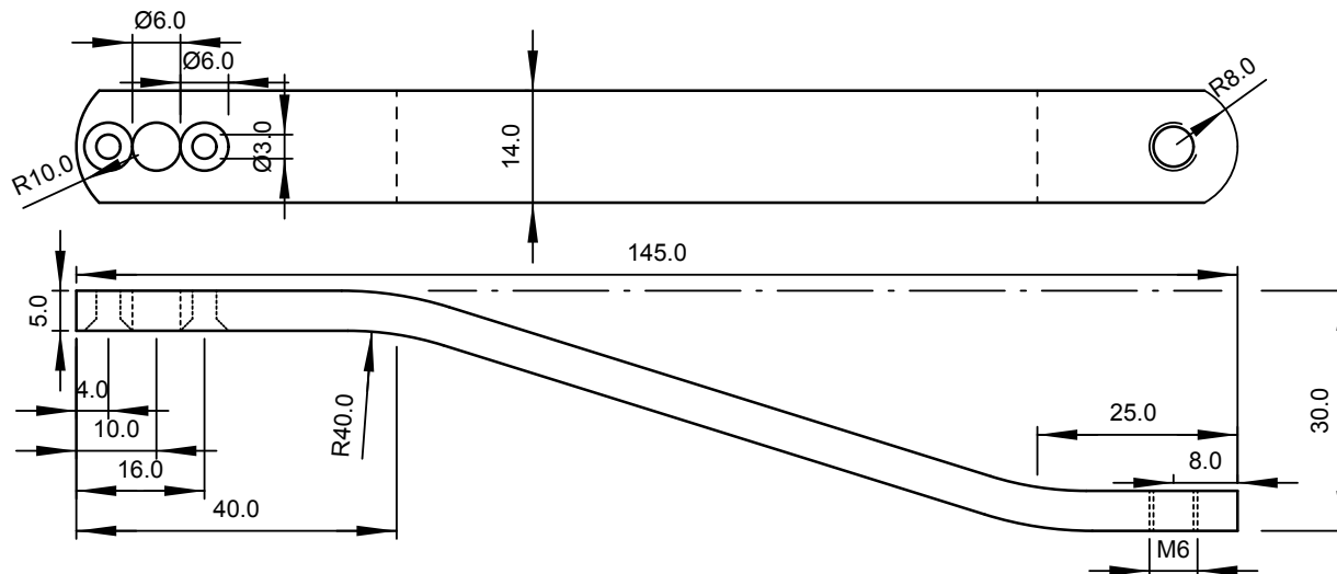
Kurbelarm, Stahl (1x)
