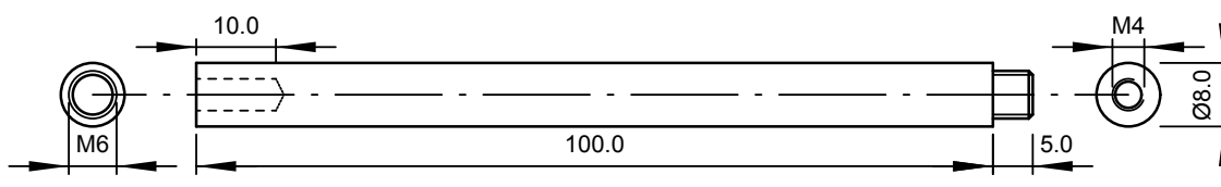
Welle Kurbelgriff, Stahl (1x)
