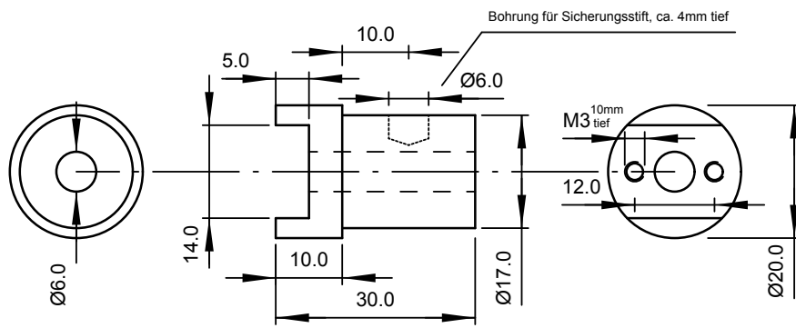
Kurbelaufnahme, Stahl (1x)
