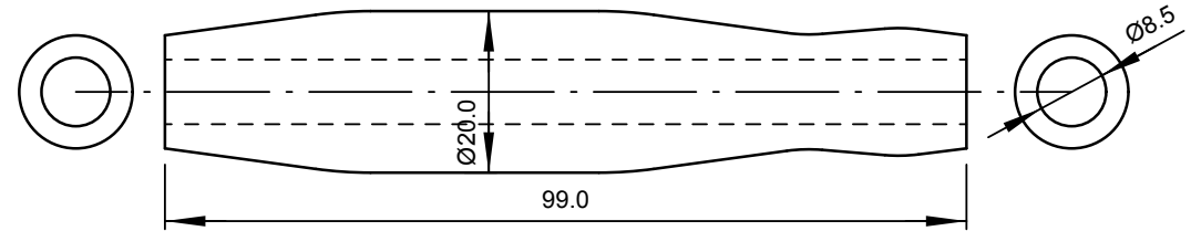
Kurbelgriff, Hartholz (1x)
