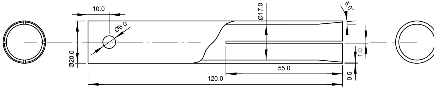
Klemmhülse, Stahl (1x)
