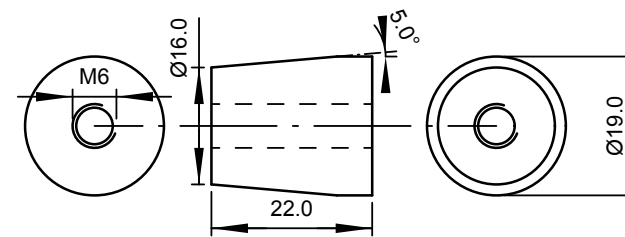
Spreizbolzen, Stahl (1x)
